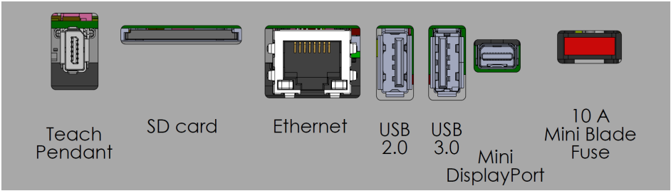
Ports de connexion externes.
