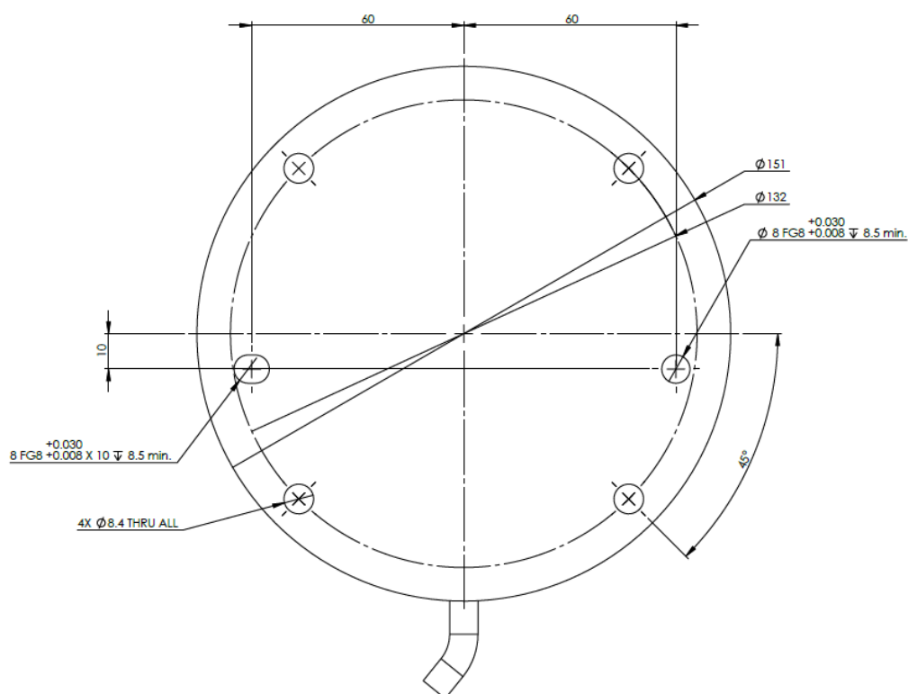
1.1: Vue de dessous de la base du robot
